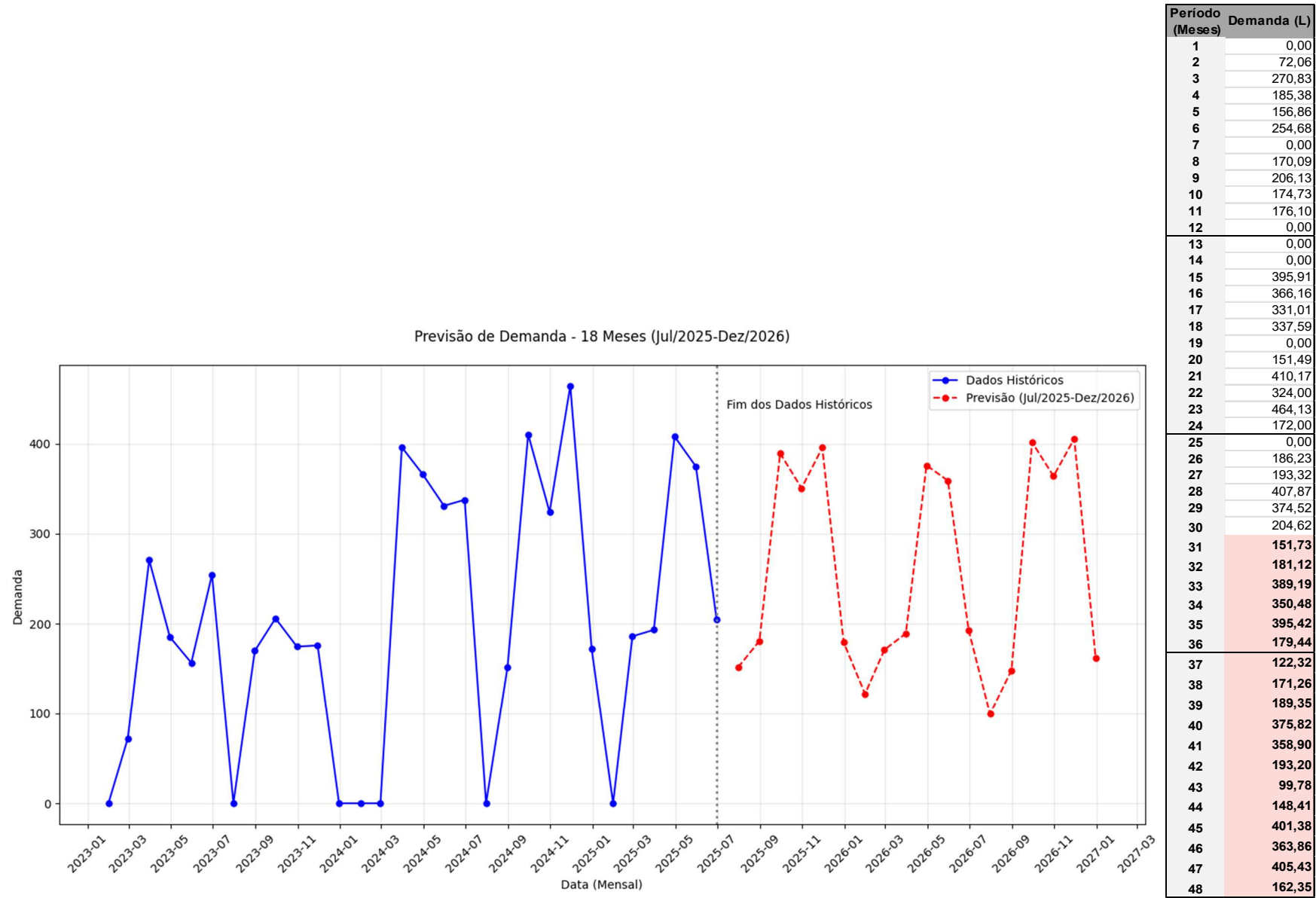
Gráfico 12- Previsão Veículo 11
